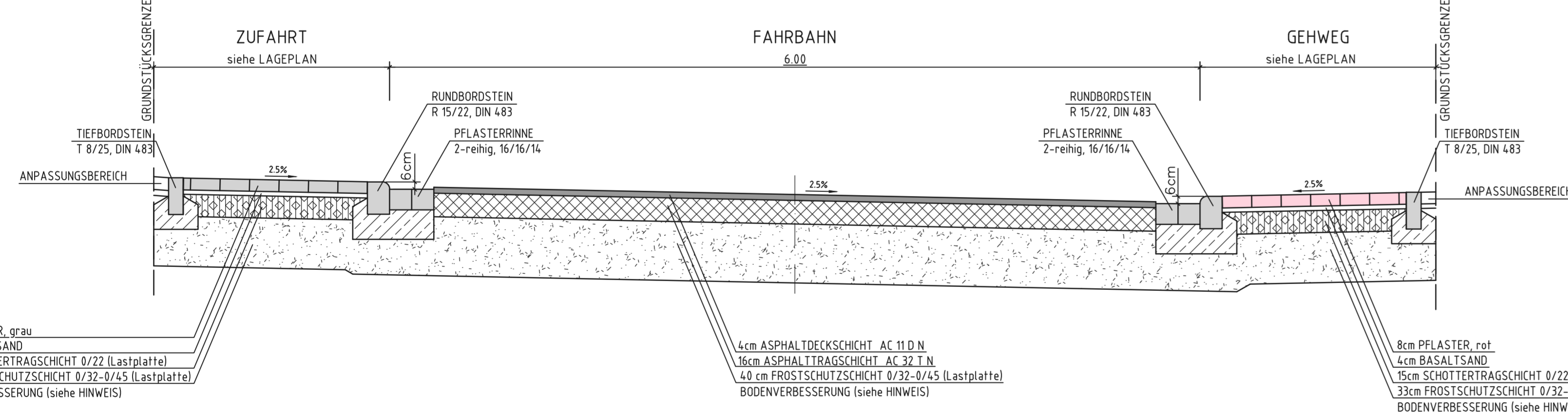
SCHNITT C-C REGELPROFIL mit Bankett 1:25
