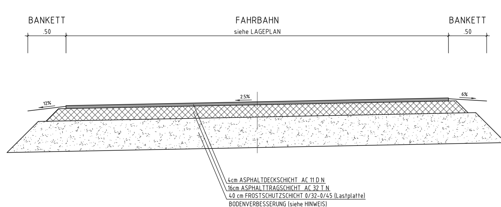
SCHNITT C-C REGELPROFIL mit Bankett 1:25
