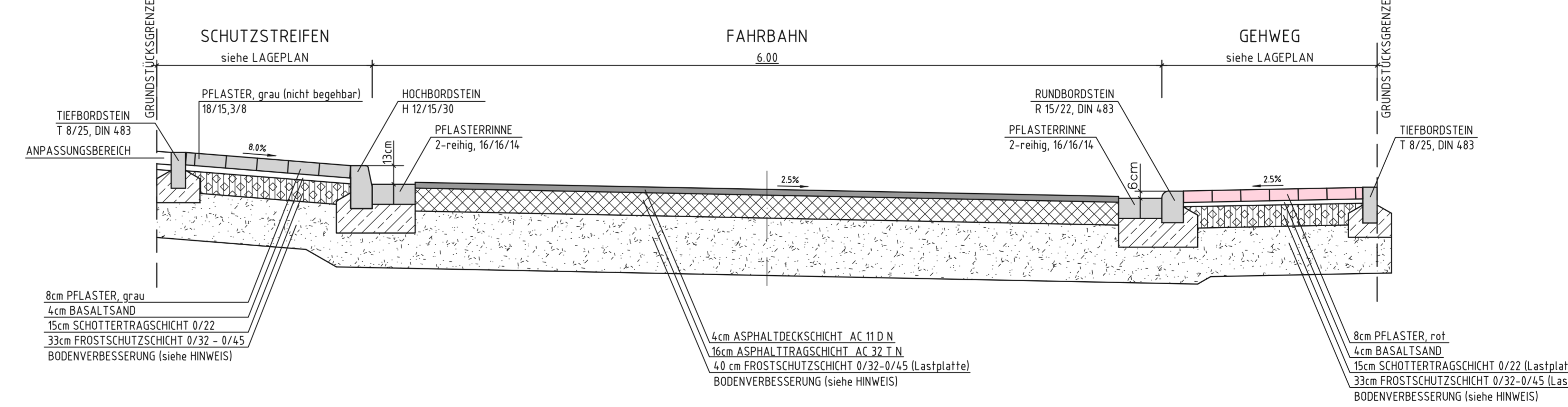
SCHNITT A-A REGELPROFIL ohne Zufahrt 1:25
